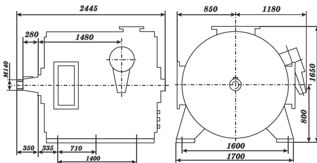
Рисунок 1. Габаритные, установочные и присоединительные размеры двигателя АКДЭ-16-62-10
